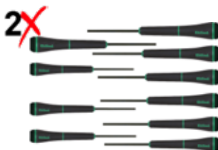
92200 Set surubelnite TORX cu cap rotitor pentru electronisti 10 piese: T3, T4, T5, T6, T7, T8, T9, T10, T15
