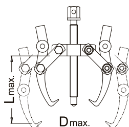
980P2 Support metalic pentru extractoare cu doua brate (612653)
